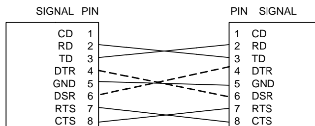
Figure 3. 시리얼 케이블
