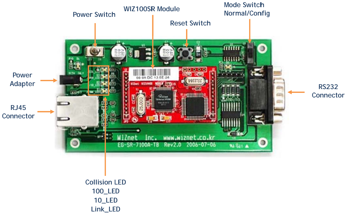
Figure 1. WIZ100SR 테스트보드
