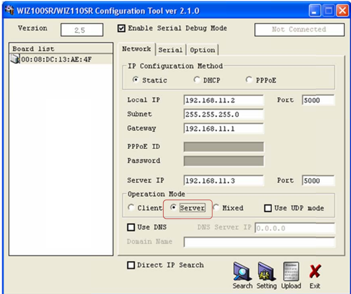
Figure 11. Password 설정을 위한 Operation Mode 선택
