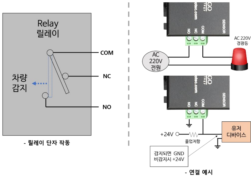
그림 4. 외부 기기의 연결 (예시)
