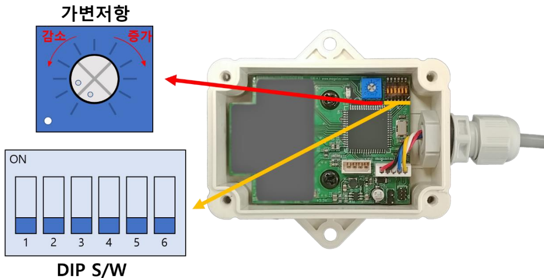
그림 5. CARDET-101 센서의 설정 스위치(좌측 그림은 기본값)
