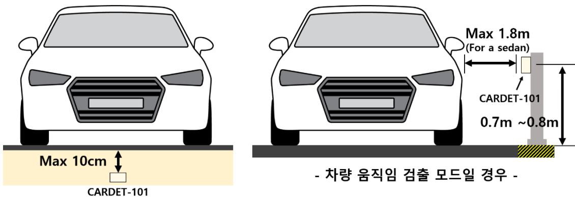
그림 1. 차량감지센서 CARDET-101의 설치
