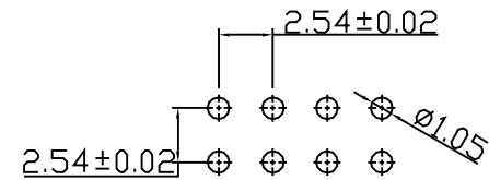
P.C.Board Layout
