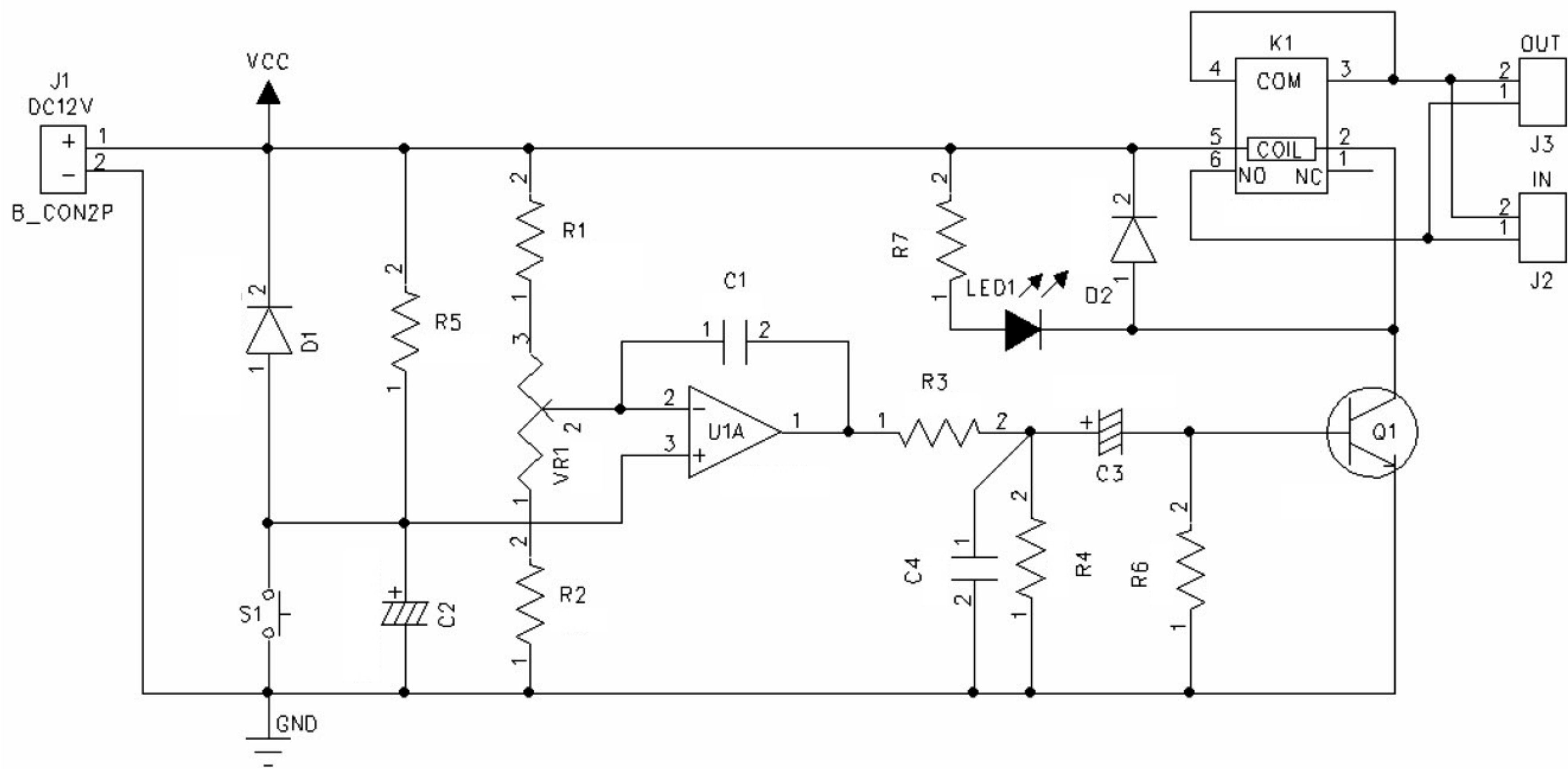
FK-5107 회로도
