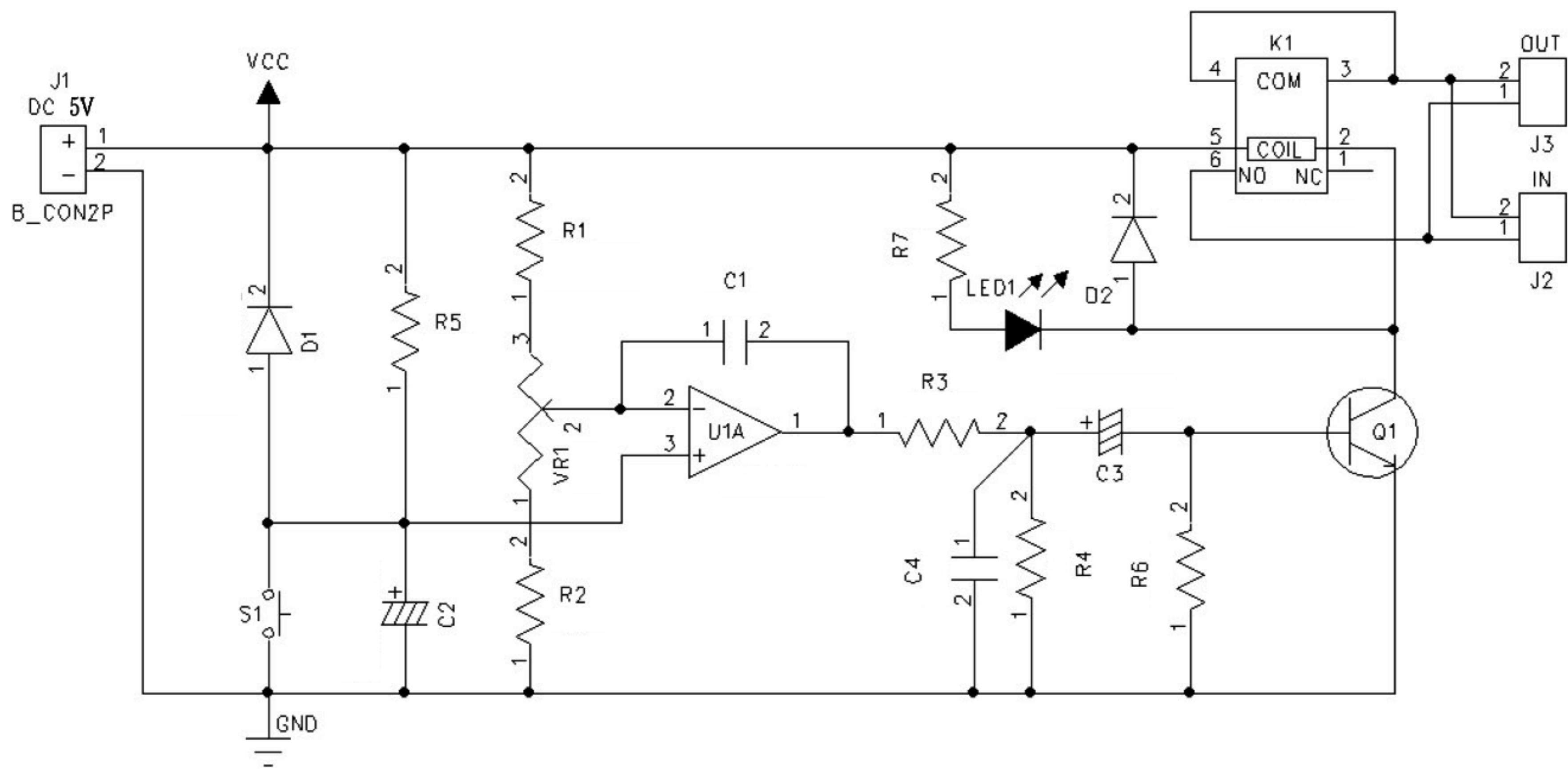
FK-5106 회로도
